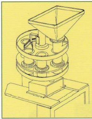
Dosatore volumetrico Doseur volumétrique Volumetric doser
