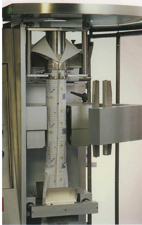
Dosatore a coclea Doseur à vis Augers fillers
